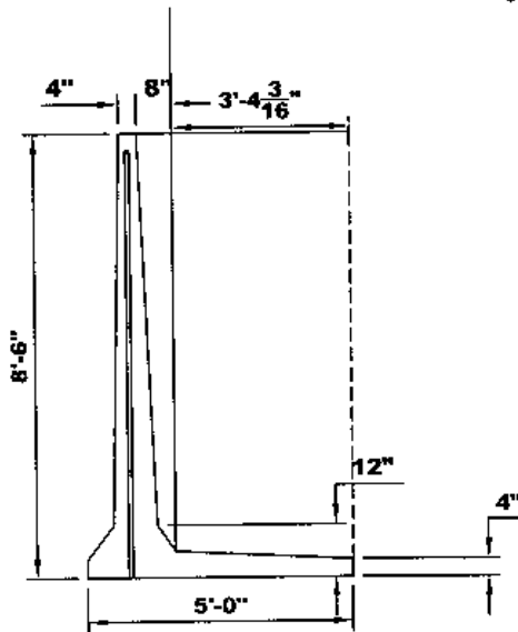
SIDE ELEV.
